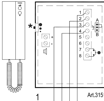
Posizione ponticello mobile JP1 Jumper JP1 position
